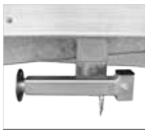
Možnost podpěrných noh pro fixaci přívěsu při nakládání
